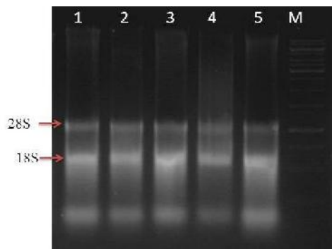
شکل ۶- الکتروفورز RNA استخراج شده از گیاهان تراریخته لاین ۱ الی ۴، ۵: RNA استخراجی از توتون شاهد (غیر تراریخته) M: مارکر ۱Kb
