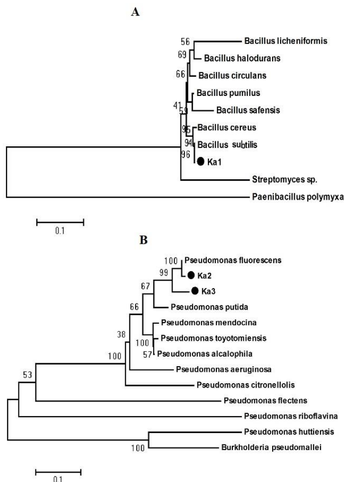
شکل ۵- A- درخت فیلوژنتیکی حاصل از مقایسه ژن 16S rRNA جدایه Ka1 جداشده از ریزوسفر گوجه‌فرنگی با سایر باکتری‌های موجود در NCBI و B- درخت فیلوژنتیکی حاصل از مقایسه ژن 16S rRNA جدایه‌های Ka2 و Ka3 جداشده از ریزوسفر گوجه‌فرنگی با سایر باکتری‌های موجود در NCBI با استفاده از نرم‌افزار MEGA5
