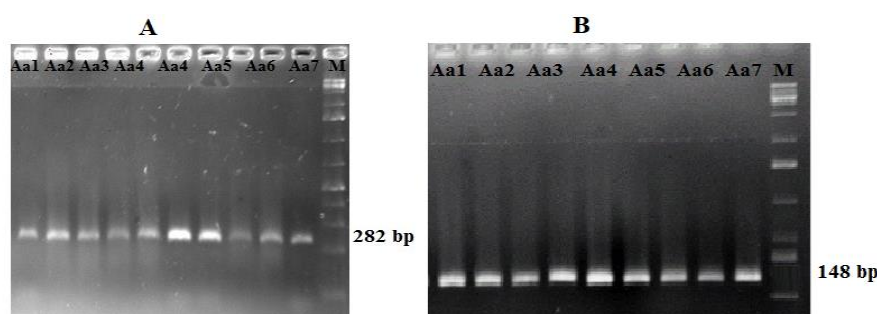
شکل ۲ - A- قطعه ۲۸۲ بازی تکثیر شده جدایه‌های R. solanacearum (Aa1 تا Aa7) با استفاده از آغازگرهای ۷۵۹/۷۶۰/B- قطعه ۱۴۸ بازی تکثیر شده جدایه‌های R. solanacearum (Aa1 تا Aa7) با استفاده از آغازگرهای PS96I/ PS96H، در ژل آگار ۱/۵ درصد رنگ‌آمیزی شده با اتیدیوم بروماید.
