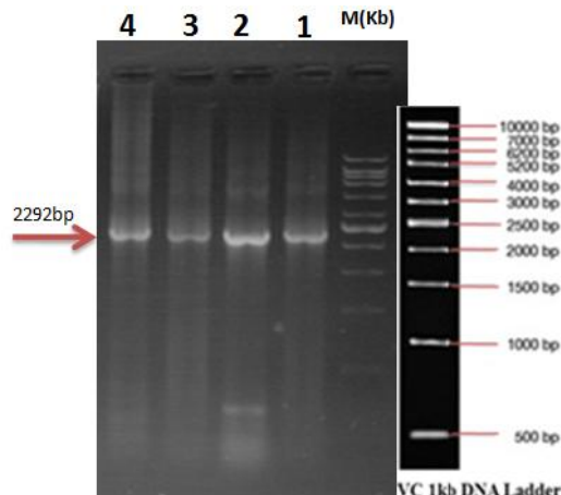
شکل ۵- تصویر الکتروفورز محصول PCR حاصل از بررسی تعدادی از پلاسمیدهای نوترکیب استخراج شده، با استفاده از جفت آغازگر اختصاصی ژن RGT2 . مشاهده باند ۲۲۹۲bp حضور قطعه همسانه‌سازی شده در کلونی‌ها را تایید می‌کند. ۱، ۲، ۳ و ۴ چهار تکرار مستقل هستند. M(Kb) مارکر.
