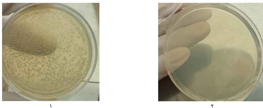
شکل ۵- پلیت ۱: کلنی های حاصل از ترانسفورماسیون روی محیط کشت جامد حاوی اسپکتینومایسین؛ پلیت ۲: کنترل منفی.
