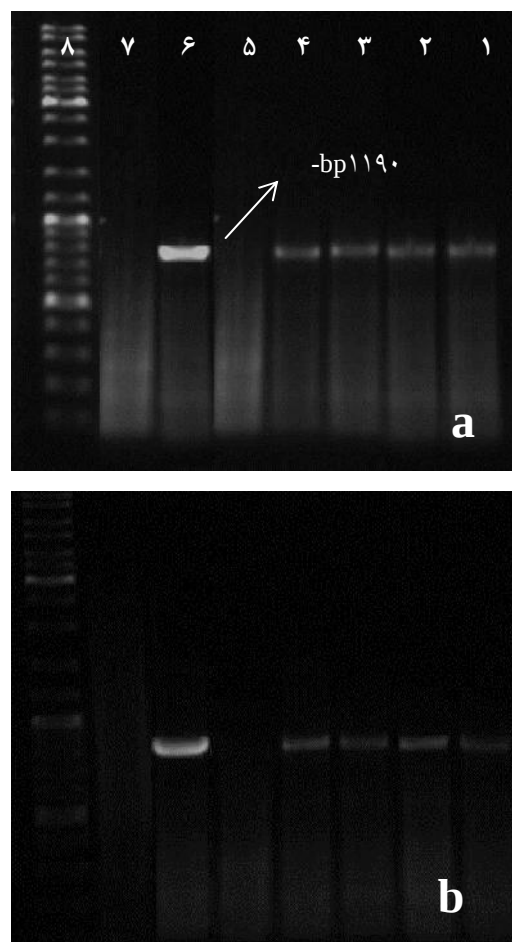
شکل ۲: نتایج PCR برای تشخیص ژن cry1Ab در نمونه‌های برگ (a) و غده (b). ۱- کنترل منفی (آب)، ۲- کنترل مثبت (پلاسمید)، ۳- کنترل منفی (گیاه غیرتراریخته) ۴-۷- گیاهان تراریخته.
