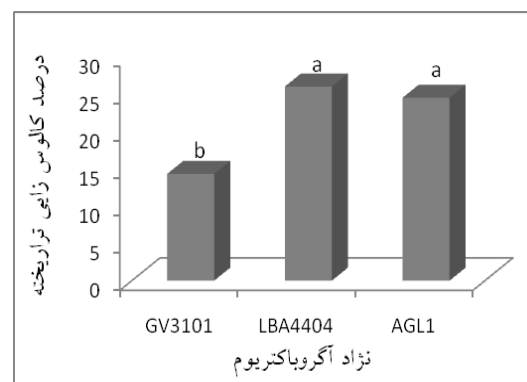
شکل ۳- مقایسه میانگین کارایی سویه‌های مختلف آگروباکتریوم در تراریزش گیاه جو.
