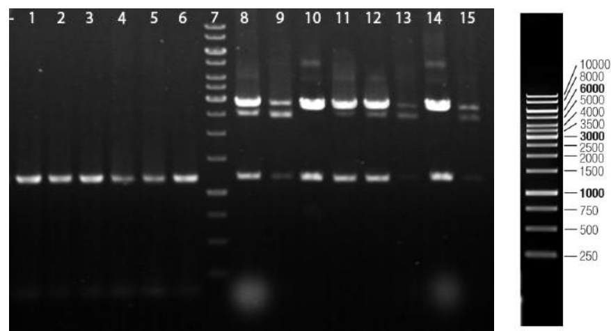
شکل ۲- الکتروفورز محصولات RT-PCR با استفاده از آغازگرهای ZYMV-8407-s و ZY3 (راهک‌های ۱ تا ۶) و پلاسمیدهای نوترکیب حاوی ZYMV-CP ناحیه (راهک ۸ تا ۱۵) در ژل آگارز یک درصد. راهک ۷: مارکر GeneRuler 1 kb DNA Ladder.
