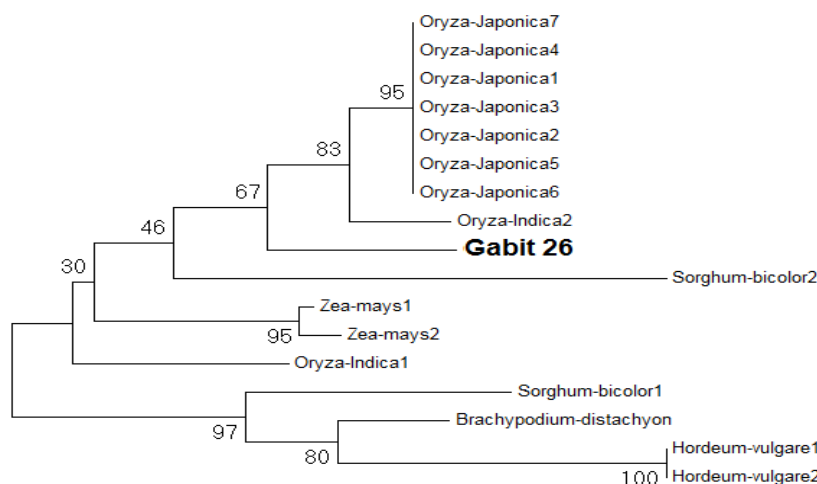
شکل ۴- نمایش درخت فیلوژنتیکی پروتئین‌های موجود در پایگاه داده‌ها (نتایج حاصل از BlastX) به همراه (JZ191067.1) با استفاده از برنامه Clustal W، MEGA 5 و الگوریتم NJ.
