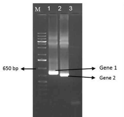
شکل ۵- محصول PCR پلاسمیدهای نو ترکیب با استفاده از آغازگرهای M13. چاهک ۱ مربوط به پلاسمید نو ترکیب حاوی قطعه ۶۳۳، چاهک ۲ مربوط به پلاسمید نو ترکیب حاوی قطعه ۵۴۴ جفت بازی و چاهک ۳ به عنوان کنترل منفی آزمایش (آب) است.
