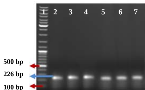
شکل ۱- شناسایی ژن اینورتاز در ژنوم نمونه‌های ذرت مورد بررسی با استفاده از جفت آغازگر IVR1-F/ IVR2-R. ۱. نشانگر اندازه ۱۰۰ bp، ۲. کنترل منفی از ذرت داخلی غیر تراریخته، ۳-۷. نمونه‌های ذرت وارداتی مورد آزمایش.
