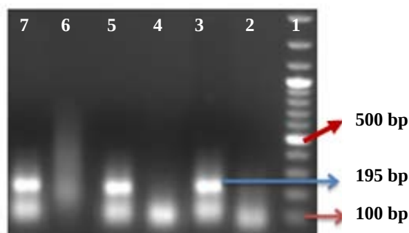
شکل ۲- شناسایی توالی پیشبر CaMV 35S در ژنوم نمونه‌های ذرت مورد بررسی با استفاده از جفت آغازگر 35S-1/35S-2. ۱. نشانگر اندازه ۱۰۰ bp، ۲. کنترل منفی از ذرت داخلی غیر تراریخته، ۳-۷. نمونه ذرت مورد آزمایش.
