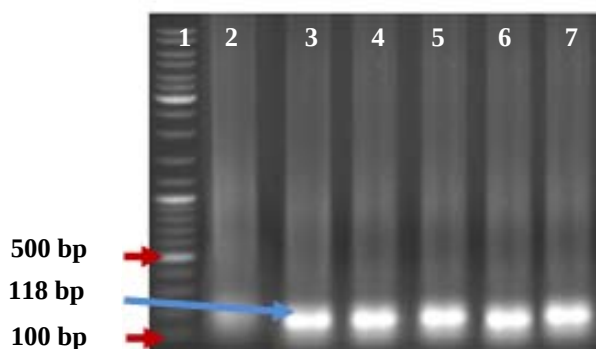
شکل ۳- شناسایی توالی پایان دهنده NOS در ژنوم نمونه‌های ذرت مورد بررسی با استفاده از جفت آغازگر HA-nos 118-f /HA-nos 118-r. ۱. نشانگر اندازه ۱۰۰ bp، ۲. کنترل منفی از ذرت داخلی غیر تراریخته، ۳-۷. نمونه ذرت‌های وارداتی.
