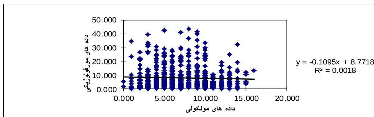
شکل ۴- نمودار آزمون مانتل با استفاده از ماتریس شباهت حاصل از داده‌های پروتئینی (پروتئین محلول در آب و نمک) و ماتریس فاصله حاصل از صفات مورفولوژیکی در ژنوتیپ‌های عدس مورد مطالعه.
