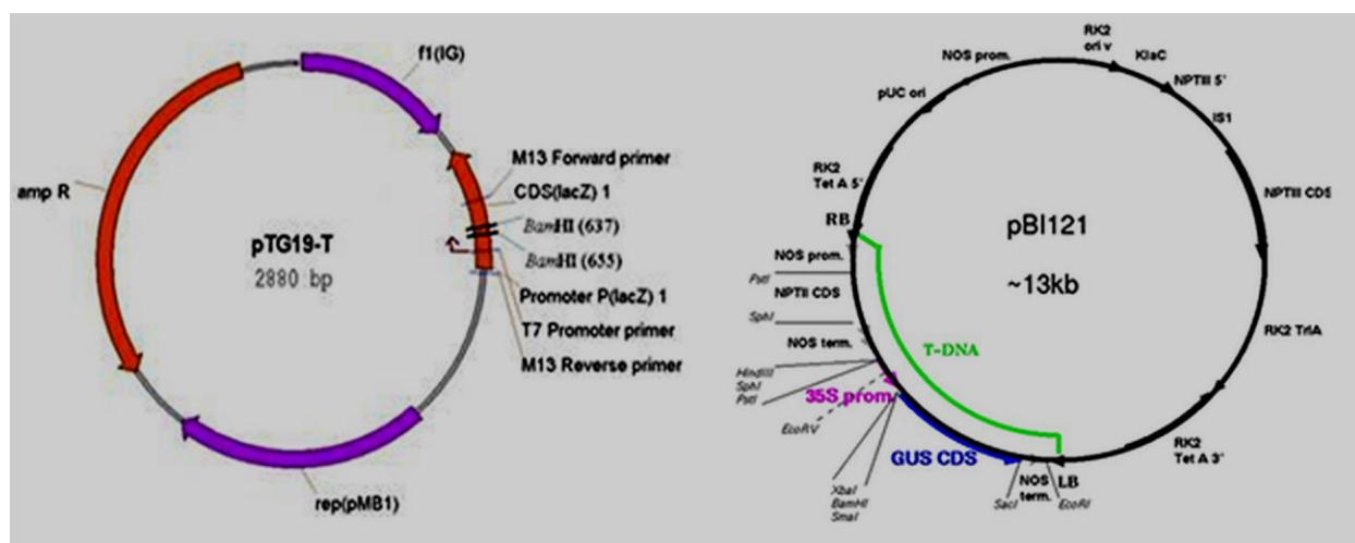
شکل ۲- ناقل های pBI121 و pTG19-T و جایگاه های برشی آنها Figure 2- pTG19-T and pBI121 vectors and their restriction sites.
