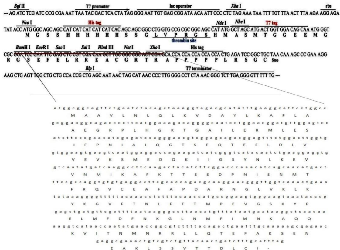
شکل ۴- محل‌های همسازگی چندگانه مربوط به پلاسمید pET28a (+) در قسمت بالا و توالی نوکلئوتیدی به دست آمده از ژن پروتئین پوششی ویروس لکه برگی کروتیک سیب جدایه SSa در قسمت پایین، که توالی ژن با قسمت مشخص شده در MCS جایگزین گردید.
