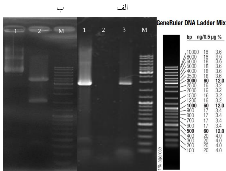
شکل ۴- الف: ۱- محصول کلنی PCR پیکیا پاستوریس نوترکیب حاوی ژن لاکاز با استفاده از آغازگرهای اختصاصی ژن لاکاز و آغازگرهای اختصاصی ناحیه پپتید نشانه alpha mating factor داخل پلاسמיד بیانی pPICZ alpha A. ۲- کنترل منفی. ۳- محصول کلونی PCR جهت شناسایی کلون‌های نوترکیب پس از ترنسفورماسیون به باکتری. M- مارکر وزنی فرمتاز (SM0333). ب: محصول هضم آنزیمی حامل بیانی pPICZ alpha A. ۱- پلاسמיד بدون هضم آنزیمی. ۲- پلاسמיד پس از هضم آنزیمی با آنزیم‌های KpnI و EcoRI. M- مارکر وزنی فرمتاز (SM0333).
