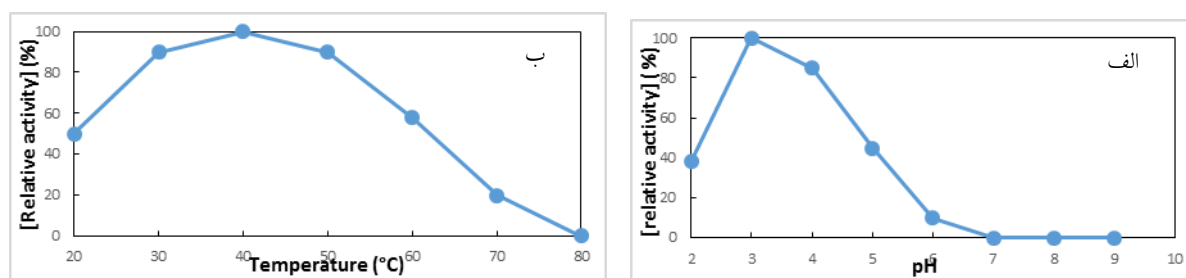
شکل ۵- الف: پروفایل فعالیت آنزیم لاکاز نوترکیب در محدوده‌ی pH ۲-۹ در دمای اتاق. ب: پروفایل فعالیت آنزیم لاکاز نوترکیب در دمای ۲۰-۸۰ درجه سانتی‌گراد.
