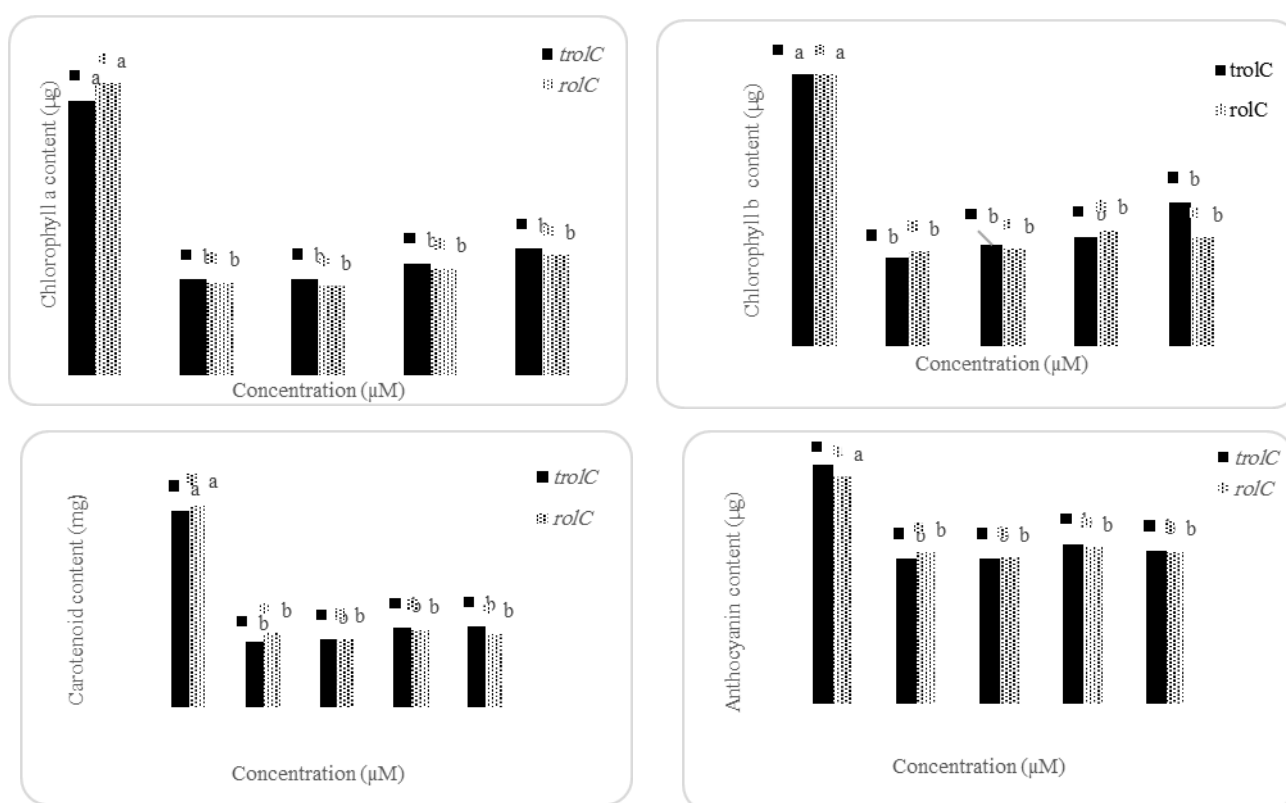
شکل ۲- محتوای رنگدانه‌ای گیاهان تراژن rolC و trlC در تیمار با غلظت‌های فزاینده دگزامتازون (dex). دگزامتازون صفر µM شرایط شاهد را نشان می‌دهد.
