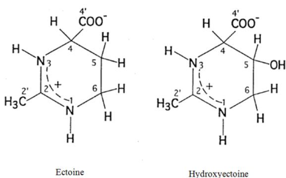
شکل ۱- ساختمان مولکولی اکتوئین و مشتق هیدروکسیله آن، هیدروکسی اکتوئین (Malin & Lapidot, 1996)
