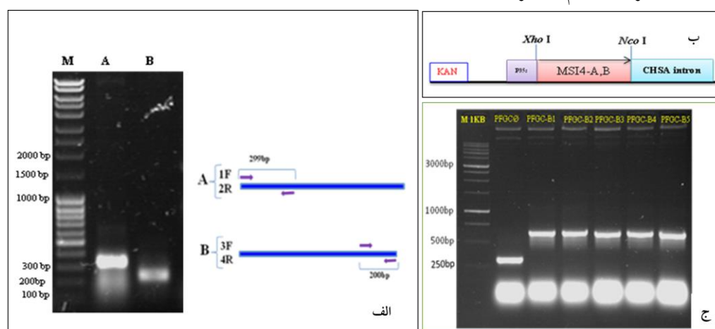
شکل ۲- الف: تصویر ژل الکتروفورس محصول PCR تکثیر ابتدا و انتهای ژن MSI4 که قطعه A ۳۰۰ جفت باز و قطعه B ۲۰۰ جفت باز است. ب: شکل شماتیک ورود قطعات سنس A و B قبل از ایترون و بعد از راه انداز. ج: تصویر ژل الکتروفورس محصول PCR تایید کلونینگ قطعه B در جهت سنس با پرایمرهای روی پلاسمید. چاهک کنار مارکر پلاسمید خالی و چاهک‌های بعدی PCR از استخراج پلاسمید نو ترکیب حاوی قطعه B را نشان می‌دهد.
