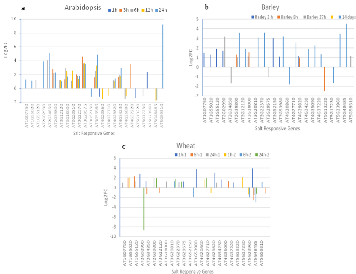
شکل ۲- سطح بیان نسبی ژن‌های حفاظت شده پاسخ دهنده به شوری در گونه‌های آرابیدوپسیس (a)، جو (b) و گندم (c) بر اساس داده‌های ریزآرایه. سطح بیان نسبی بر حسب \text{Log}_2\text{FC} آرایه شده است.
