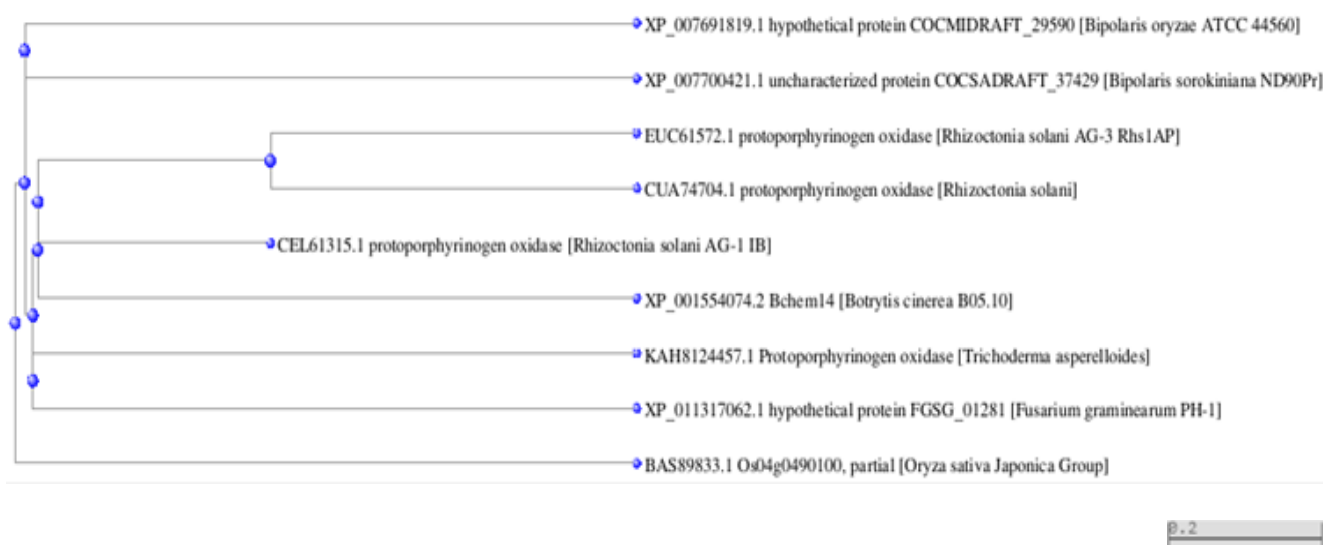
شکل ۳- درخت همدیف‌سازی کوبالت توالی‌های پروتوپورفیرینوژن اُکسیداز قارچ‌های Fusarium , Botrytis cinerea , Bipolaris sp. و Oryza sativa Japonica از Trichoderma asperelloides و Rhizoctonia solani در همسنجی با برون‌گروه گروه Japonica از Oryza sativa Fig. 3. The COBALT alignment tree of protoporphyrinogen oxidase sequences from the fungi Bipolaris sp., Botrytis cinerea , Fusarium graminearum , Rhizoctonia solani , and Trichoderma asperelloides as compared to that from the outgroup, Oryza sativa Japonica group
