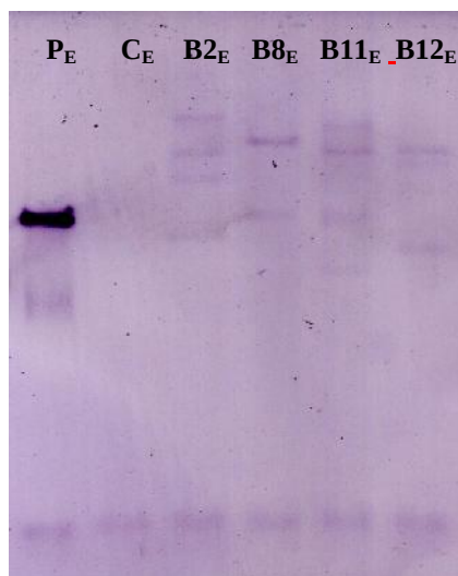
شکل ۳: تجزیه و تحلیل سادرن گیاهان تراریخته سیبزمینی حاوی ژن cry1Ab . PE، پلاسمید هضم شده با آنزیم EcoRI ; C E ، گیاه غیرتراریخته هضم شده با آنزیم EcoRI ; B2 E ، B8 E ، B11 E ، B12 E ، DNA تراریخته هضم شده با آنزیم EcoRI .
